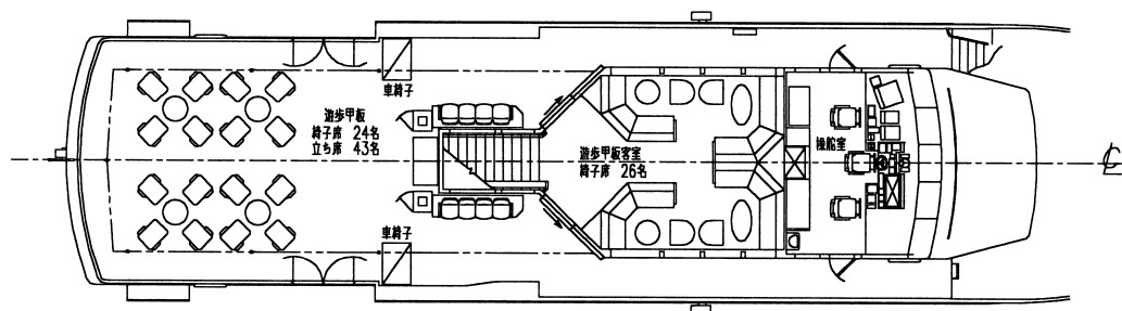
遊歩甲板
