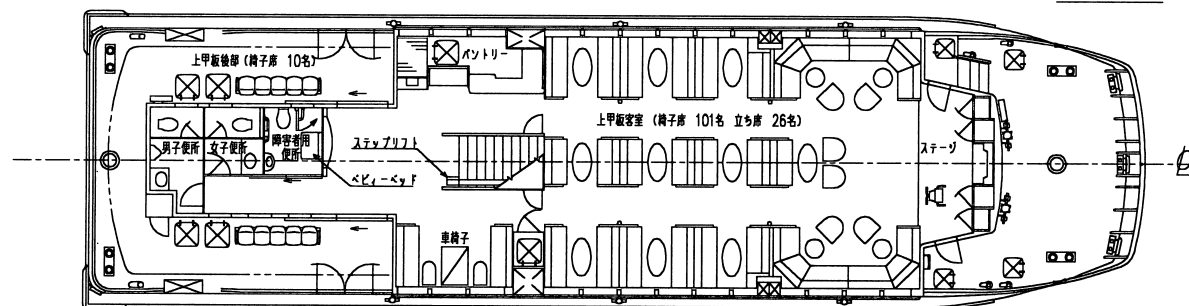
上甲板
